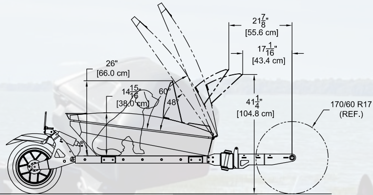
Remorque équipée d'un coffre haut de gamme fermé en aluminium avec option chien
