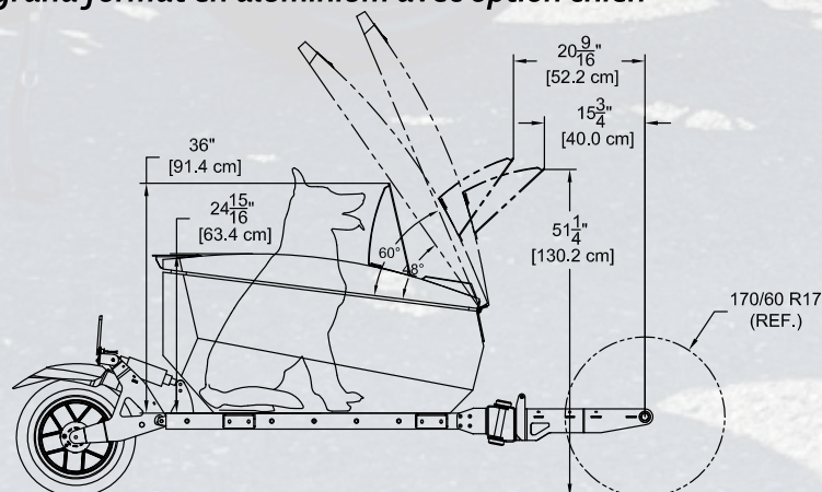
Remorque équipée d'un coffre haut de gamme fermé grand format en aluminium avec option chien
