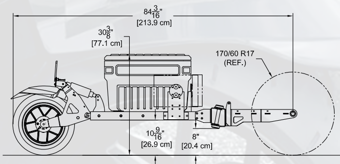
Remorque courte équipée d'un bac de plastique 90L
